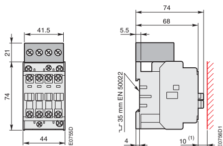
A 9, A 16, N + реле сопряжения RA 5
