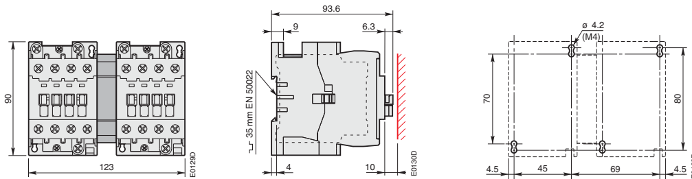
A 26 + реверсивная механическая блокировка VM 5-1
