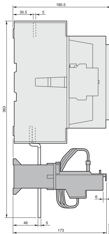
А 210, А 260, А 300, AF 210, AF 260, AF 300 с 1 x CAL 18 + блок расширения контактов LW 300
