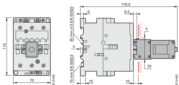
А 50, А 63, А 75, АF 50, АF 63, АF 75 + механическая защелка WB 75-А
