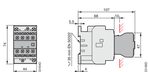
А 9, А 12, А 16 + 4-полюсный блок вспомогательных контактов фронтальной установки CA 5
