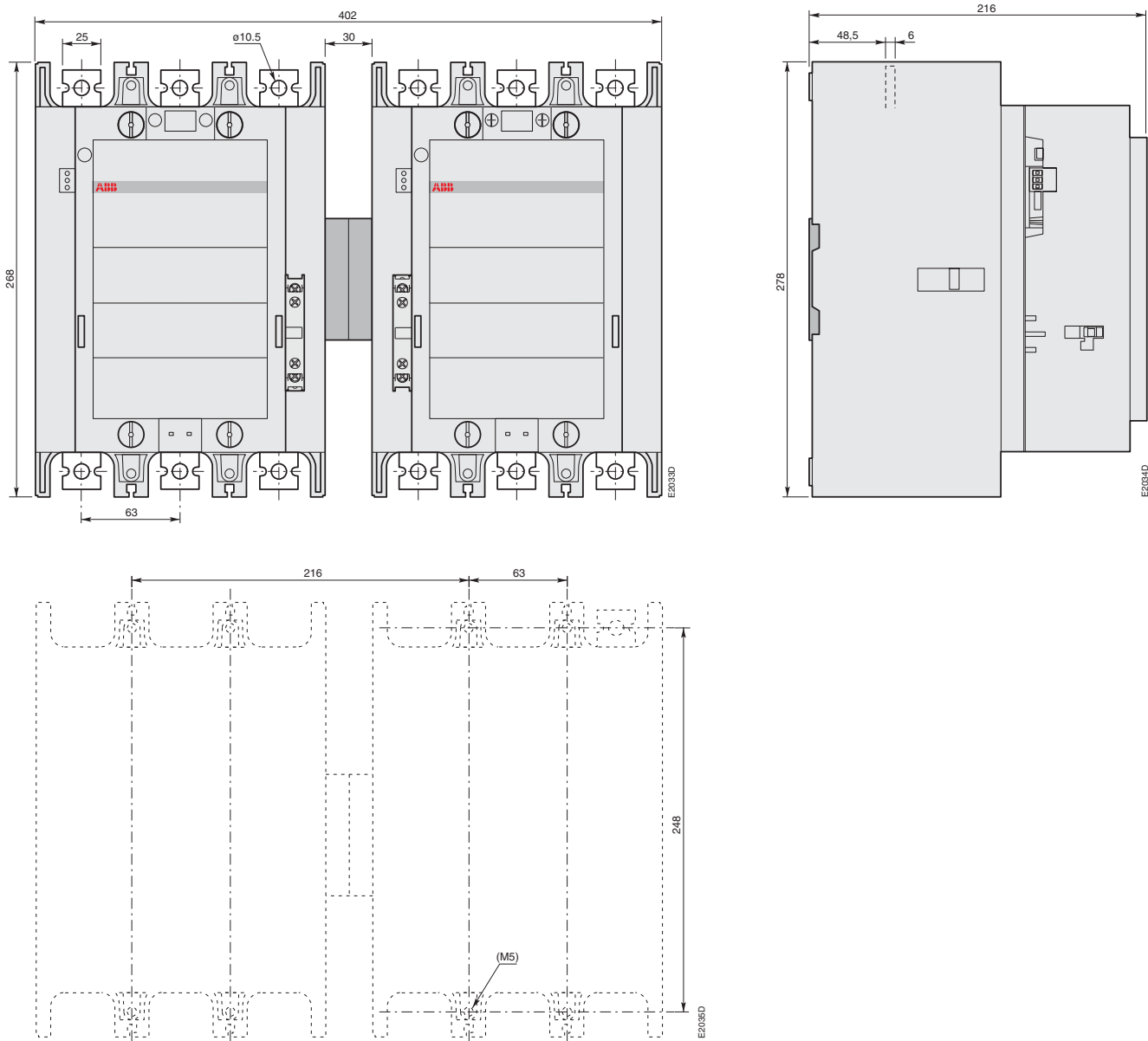
AF 400, AF 460 с 1 x CAL 18 + реверсивная механическая блокировка VM 750H
