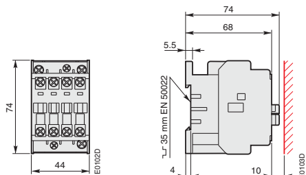
А 9, А 12, А 16
