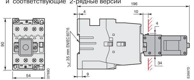
AL 30, AL 40, TAL 30, TAL 40 + WB 75-A с защелкой
