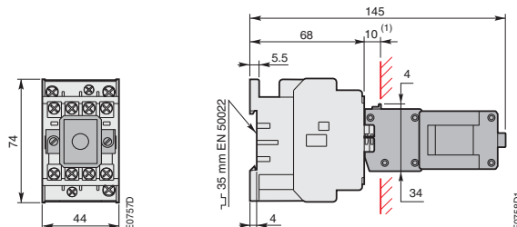
A 9, A 16, N + механическая защелка WB 75-A
