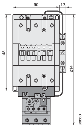
(Т) АЕ 95, АЕ 110, ТАЕ 95, ТАЕ 110 + тепловое реле ТА 80 DU
