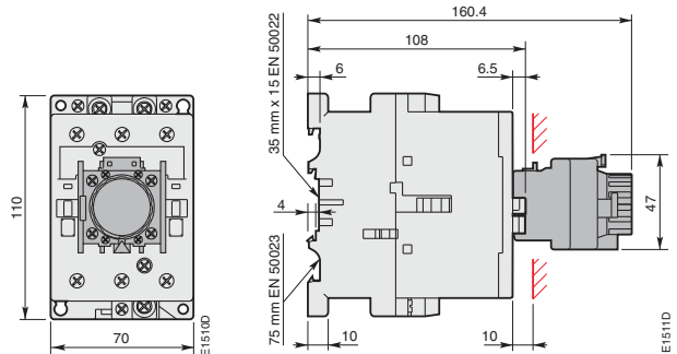
А 50, А 63, А 75, АF 50, АF 63, АF 75 + Пневматическое реле времени TP
