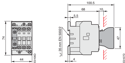
А 9, А 12, А 16 + 1-полюсный блок вспомогательных контактов фронтальной установки CA 5
