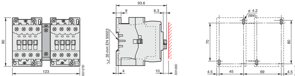
A 26 + реверсивная электрическая и механическая блокировка VE 5-1
