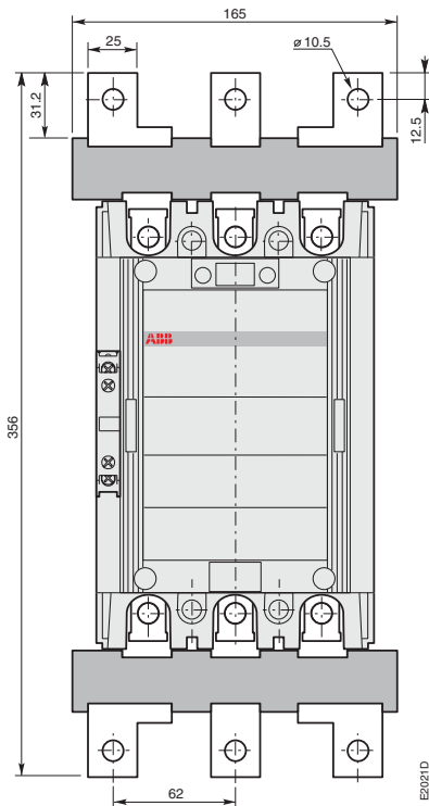
А 210, А 260, А 300, AF 210, AF 260, AF 300 с 1 x CAL 18 + блок расширения контактов LW 300
