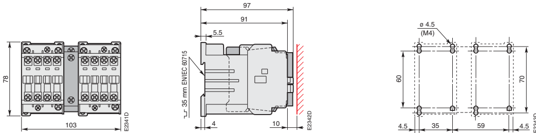
AL 9-40 ... AL 16-40 TAL 9-40 ... TAL 16-40 + VE 5-1 электрическая и механическая блокировка
