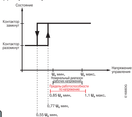
Диаграмма работы
