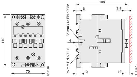
А 50, А 63, А 75, АF 50, АF 63, АF 75
