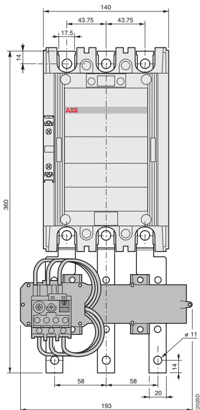
А 210, А 260, А 300, AF 210, AF 260, AF 300 с 1 x CAL 18 + тепловое реле ТА 450 DU/SU
