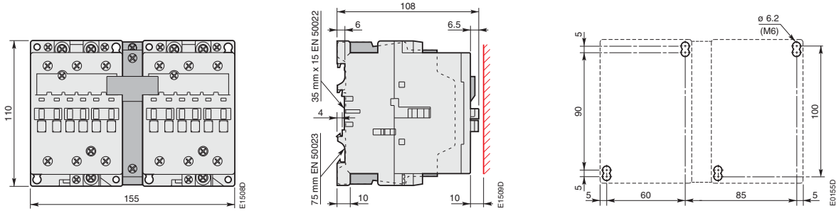
A 50, A 63, A 75, AF 50, AF 63, AF 75 + реверсивная электрическая и механическая блокировка VE 5-2
