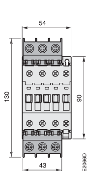
Контакты А 30, А 40, (Т) АЕ 30, (Т) АЕ 40, UA 30 + 2 x LD 40
