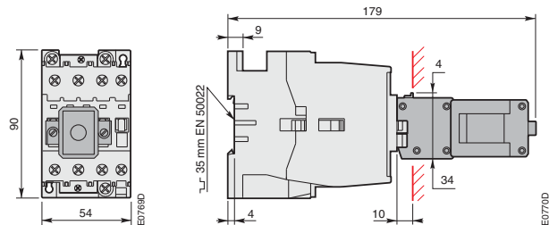
A 30, A 40 + механическая защелка WB 75-A
