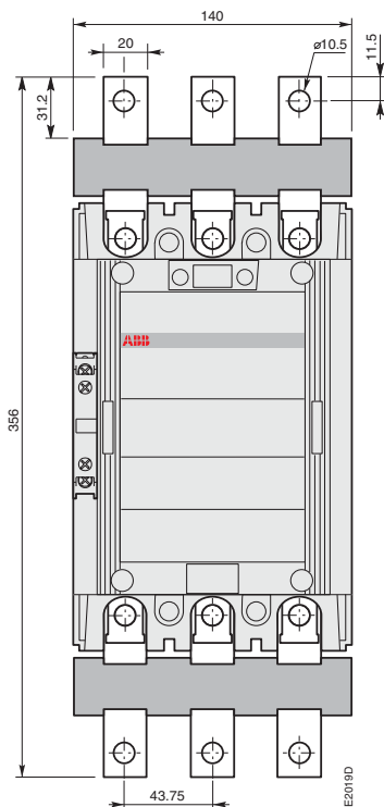
А 210, А 260, А 300, AF 210, AF 260, AF 300 с 1 x CAL 18 + блок увеличения контактов LX 300
