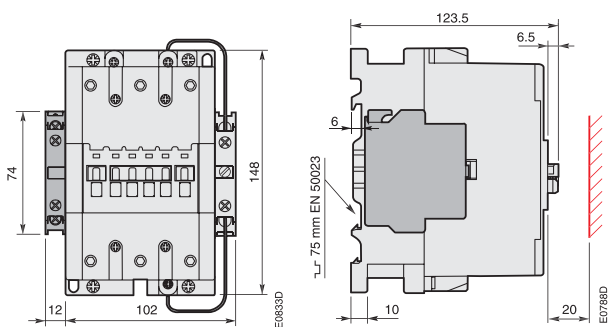
(Т) АЕ 95, АЕ 110, ТАЕ 95, ТАЕ 110 + 2-полюсный блок вспомогательных контактов боковой установки СА 18
