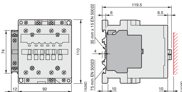
A 45, A 50, A 75, AF 45, AF 50, AF 75 + 2-полюсный блок вспомогательных контактов боковой установки CAL 5
