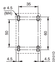
Установочные размеры для А 9, А 16, N
