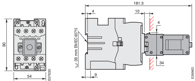
AL 26, TAL 26 + CAL 5 4-полюсный блок вспомогательных контактов для фронтальной установки и соответствующие 2-рядные версии
