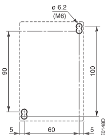
(Т) АЕ 50, АЕ 63, АЕ 75, ТАЕ 50, ТАЕ 75 + пневматическое реле времени TP
