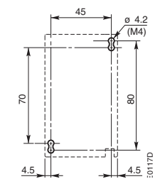
AL 30, AL 40, TAL 30, TAL 40 - Схема сверления отверстий
