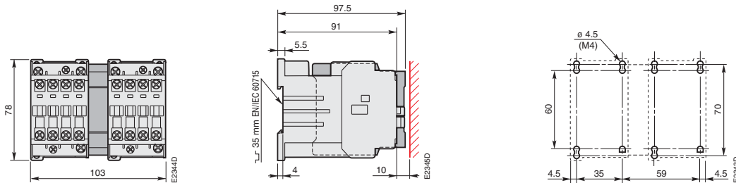
AL 9-40 ... AL 16-40 TAL 9-40 ... TAL 16-40 + VM 5-1 механическая блокировка
