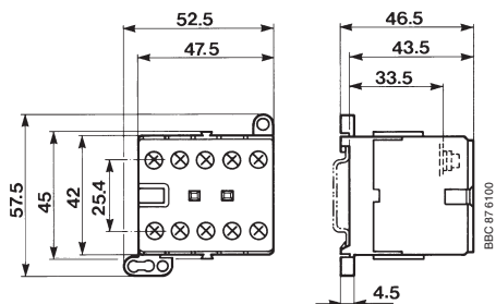
В 6, В 7, ВС 6, ВС 7, К 6, КС 6 с винтовыми зажимами соединений
